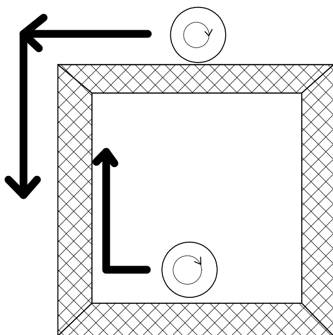
Toupillage à la main vue du dessus
